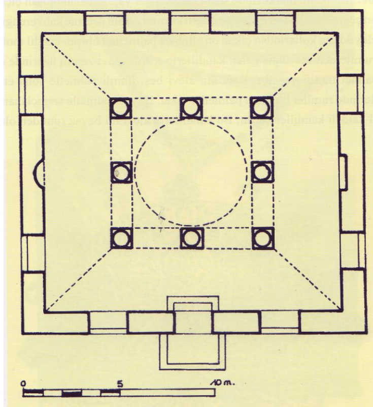
Hüdevendigâr Türbesi Planı
